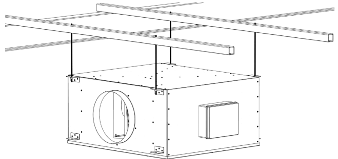
Drop Rod
