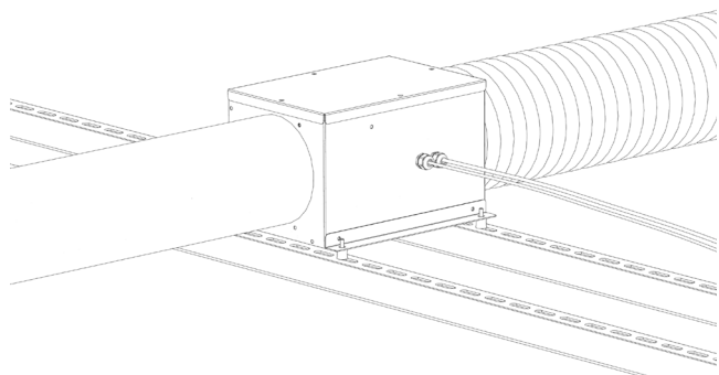
AV Mount
